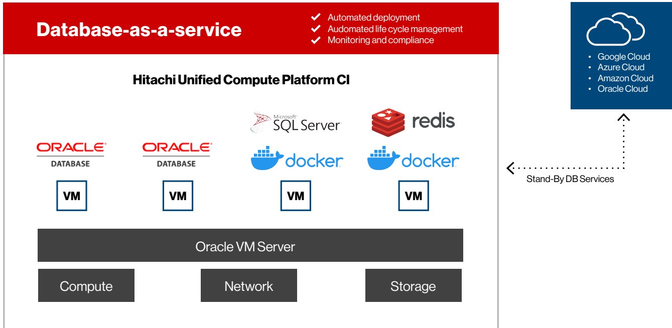
Fig.2 Database-as-a-service
